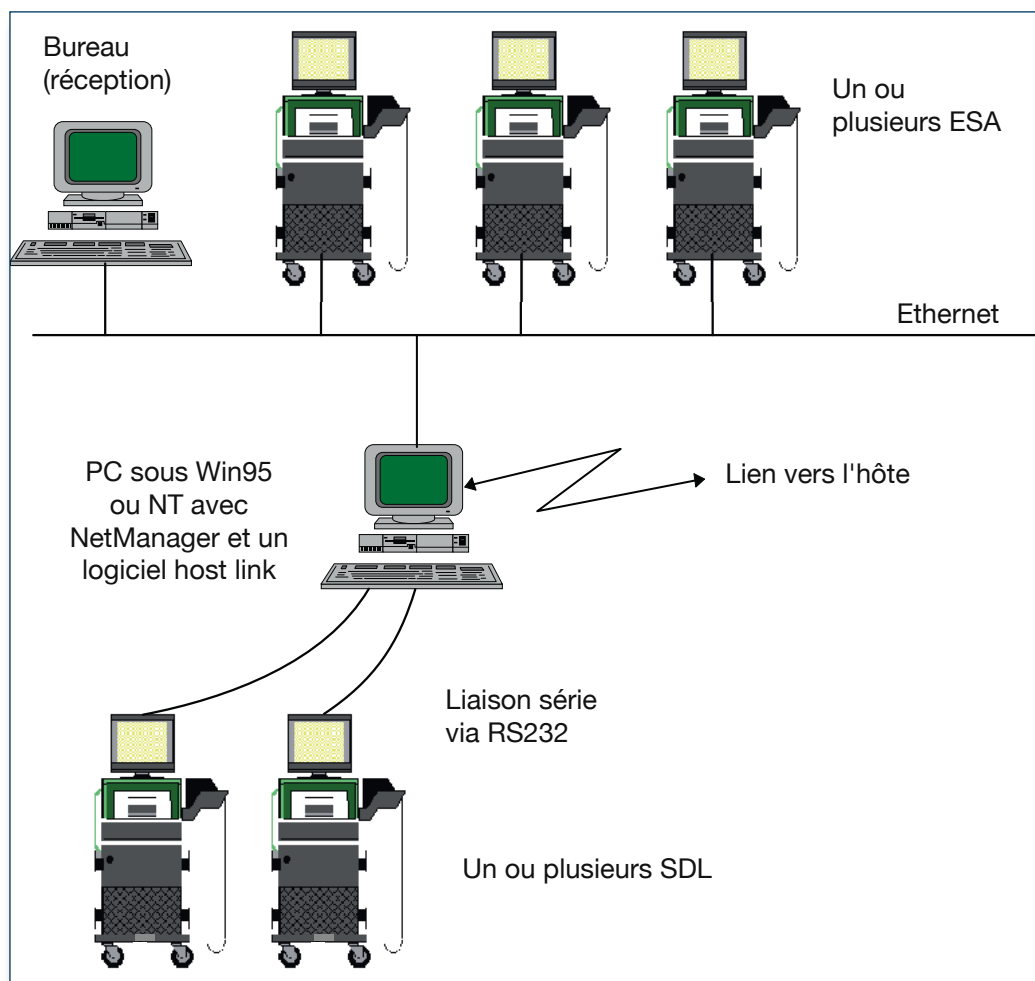
Fig. 38 Système de relevés centralisés.
