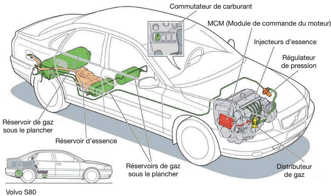
Fig. 18 Système hybride GNC. Volvo
