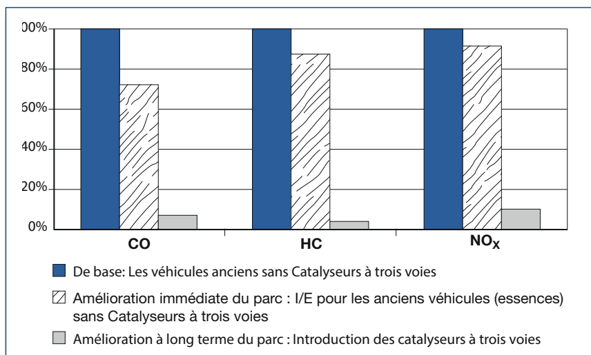
Fig. 1 Les réductions d’émissions sont possibles grâce à l’inspection et l’entretien pour les véhicules avec et sans catalyseurs à trois voies. Un système d’I/E se concentre sur les améliorations rapides de la réduction des polluants de l’air pour l’ensemble du parc automobile.
