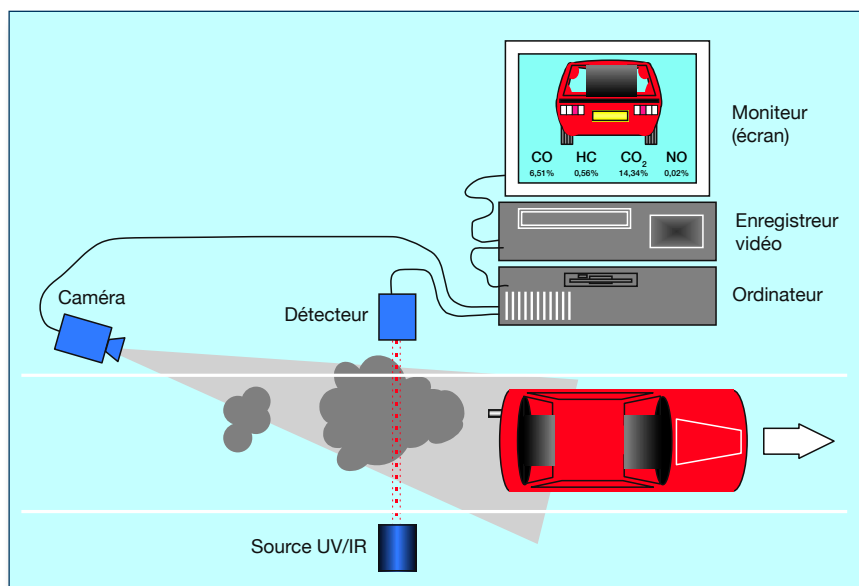
Fig. 35 Une nouvelle mesure contre les véhicules qui émettent de la fumée. http://adb.org/vehicle-emissions
